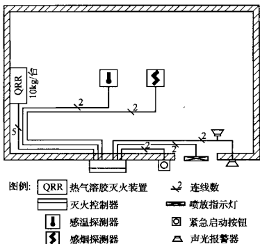
图 7 热气溶胶灭火系统
