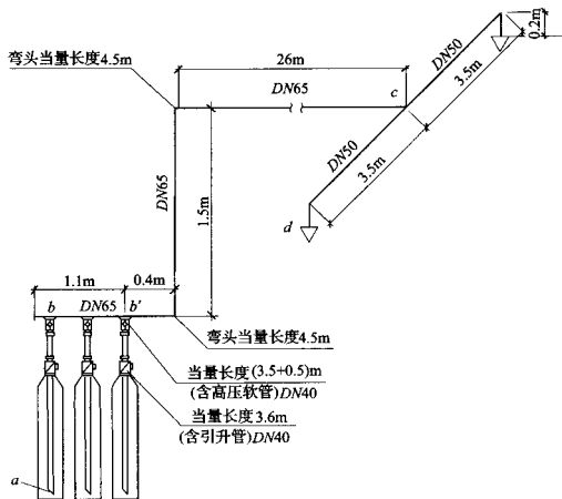
图 4 系统管网计算图
