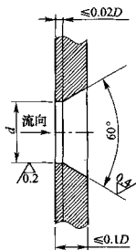
图 5 减压孔板
