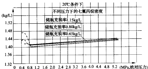
图3 不同压力下七氟丙烷的密度
