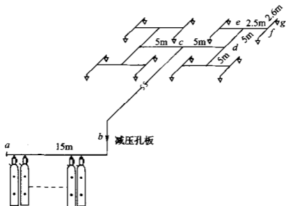
图 6 系统管网计算图
